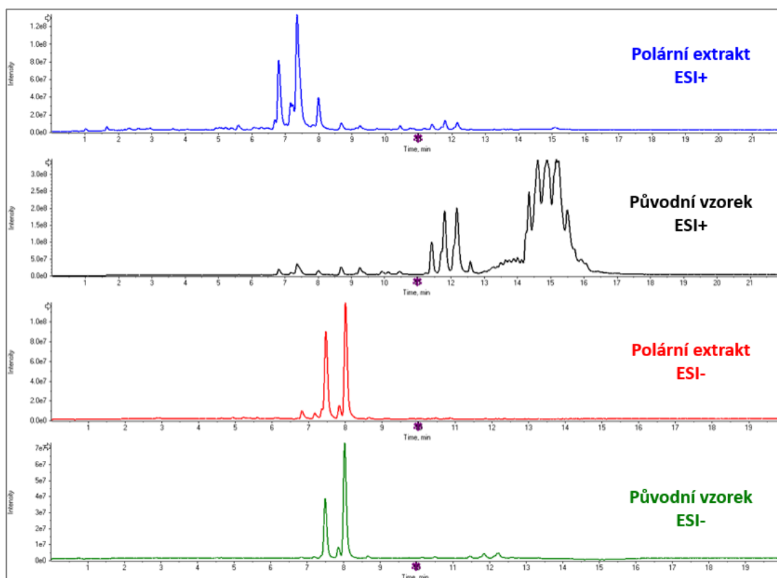
Obrázek 1: Chromatografické záznamy (metabolomické 'fingerpriny'). Modrá: MeOH:H 2 O extrakt ML 985/20, ESI+; černá: vzorek ML 985/20 naředěný ethanolem, ESI+; červená: MeOH:H 2 O extrakt ML 985/20, ESI-; zelená: vzorek ML 985/20 naředěný ethanolem, ESI-.
